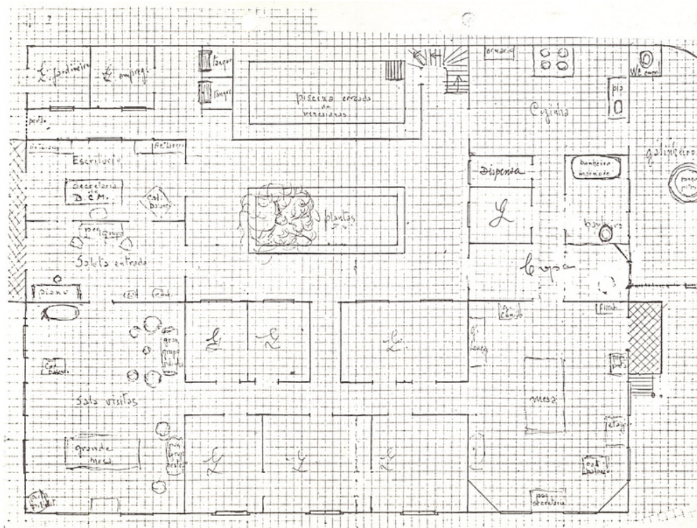
Planta baixa da casa com organização dos cômodos. Benjamin Constant de Magalhães Fraenkel. Década de 1970. Arquivo Institucional. MCBC, Ibram/MinC.
